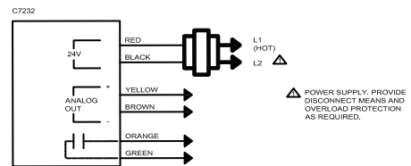
Fig. a Wiring for C7232
